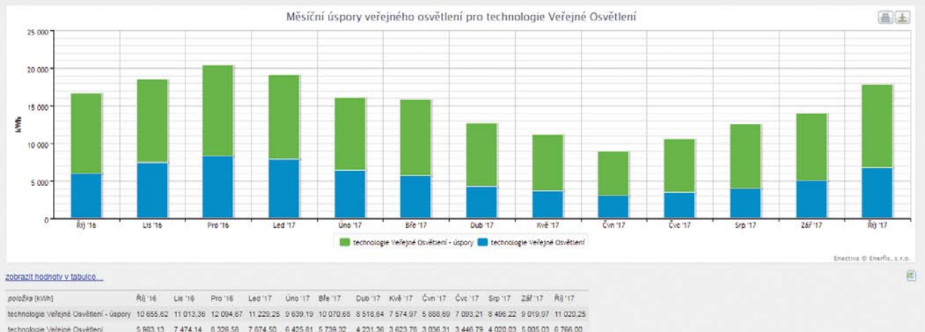
(Obrázek č. 8 - Spotřeba energií za veřejné osvětlení (celý sloupec - průměrná spotřeba v daném měsíci zprůměrovaná za roky 2014-2016, modrý sloupec - spotřeba po modernizaci VO)
